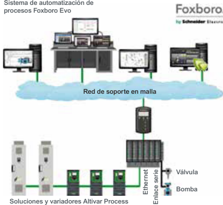
Altivar Process en la arquitectura Foxboro Evo DCS
