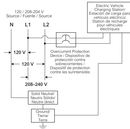
Diagrama de alambado para el cargador sencillo
